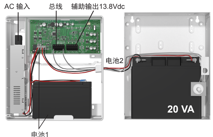
PS45 双电池组满容量后备
